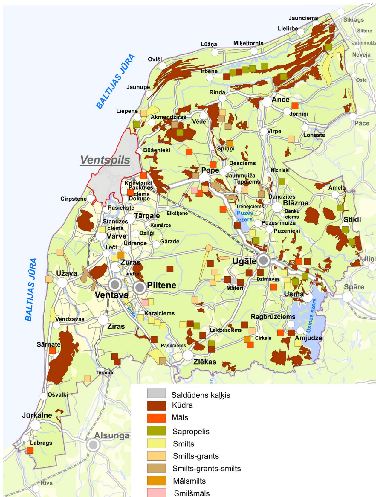
6. attēls. Derīgo izrakteņu atradnes Ventspils novadā, SIA „Reģionālie projekti” (Vita Jumtiņa), 2014. 12
